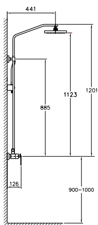
Colonne de douche - MAE500 Cartouche Ø 35 Entraxe 130 à 170 mm, rosaces, raccords excentriques, inverseur, pommeau 200 x 200 mm, douchette à main, flexible, support de flexible
