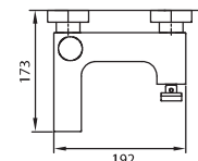
Mitigeur bain/douche - MAE33 Cartouche Ø 35 Entraxe 130 à 170 mm, rosaces, raccords excentriques, inverseur, brise-jet
