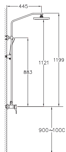
Colonne de douche - NP500 Cartouche Ø 35 Manette chromée et satinée. Entraxe 130 à 170 mm, rosaces, raccords excentriques, inverseur, pommeau 200 x 200 mm, duplex
